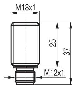
Габаритный чертеж
